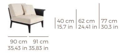
U MÓDULO RINCÓN BRAZO IZQUIERDO / CORNER MODULAR PART LEFT ARM REF.: 74243
