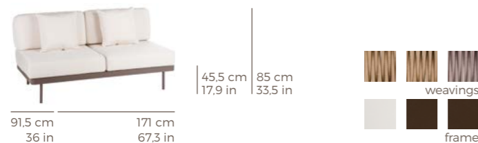
MÓDULO 2 SIN BRAZOS / MODULAR 2 WITH NO ARMS REF.: 77146
