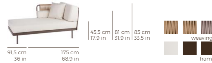
CHAISELONGUE BRAZO DERECHO / CHAISELONGUE RIGHT ARM REF.: 77196
