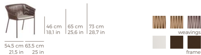
SILLÓN COMEDOR / ARMCHAIR REF.: 77107
