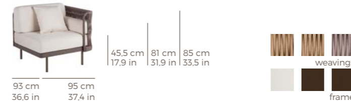
MÓDULO SILLÓN BRAZO IZQUIERDO / MODULAR ARMCHAIR LEFT ARM REF.: 77151
